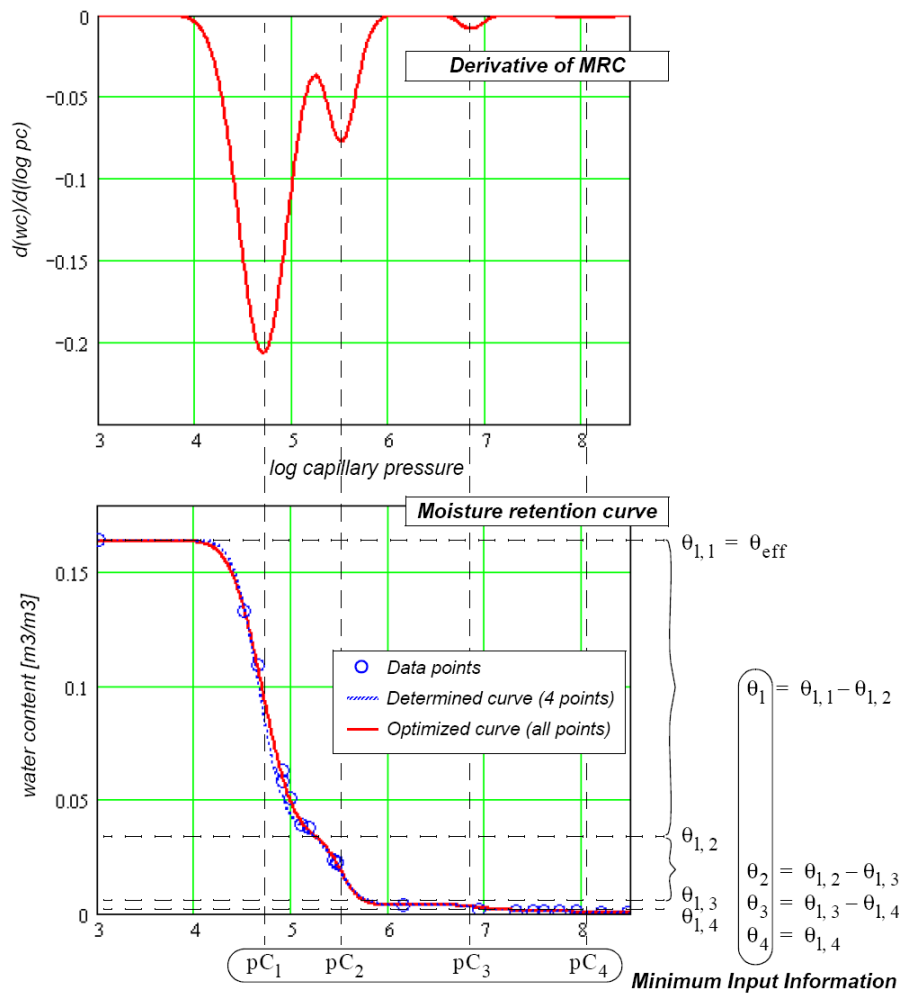
Abb. 38 Feuchtespeicher- (unten) und Porenvolumenverteilungsfunktion (oben) eines Ziegels. Die Peaks (pC) liefern die Porenradenmaxima und deren Wassergehaltsverteilungen identifizieren die korrespondierenden Porenvolumina
