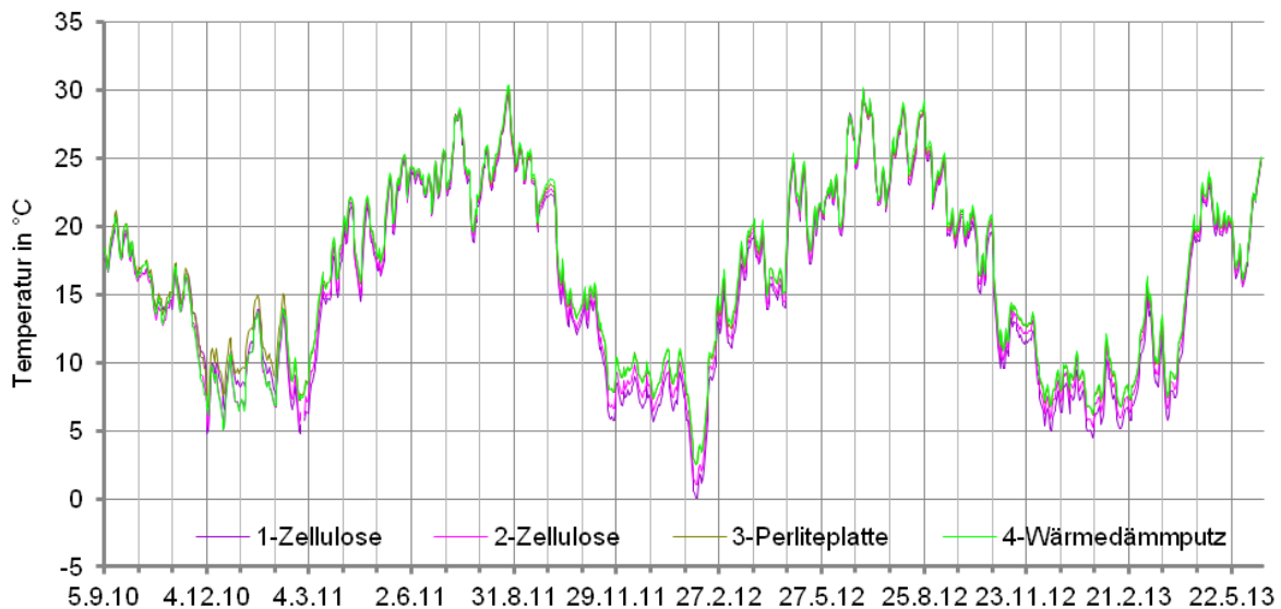
Abb. 57 Temperaturen im Luftspalt zwischen Balkenwange und Mauerwerk in ungefähr 0,15 m Entfernung von der ehemaligen Bestands- oberfläche (BA-Wa, Tageswerte): Zellulose, Perliteplatte und Wärmedämmputz
