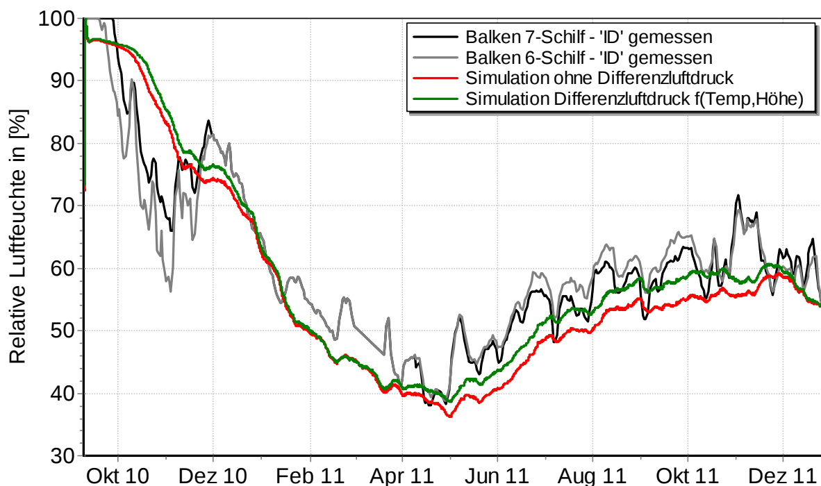
Abb. 108 Gemessene und berechnete relative Luftfeuchte (Tageswerte) für die Messposition ‚ID‘ im Feld 5 (Schilf) vom 5.9.2010 bis zum 20.12.2011
