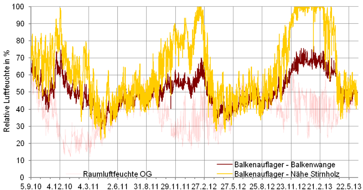
Abb. 91 Stundenwerte der relative Luftfeuchte an Balken 8: ehemalige Wandoberfläche (grün & hellblau), Balkenwange (braun), neben der Stirnfläche des Balkens (gelb) und Raumluftfeuchte im OG (rot transparent)
