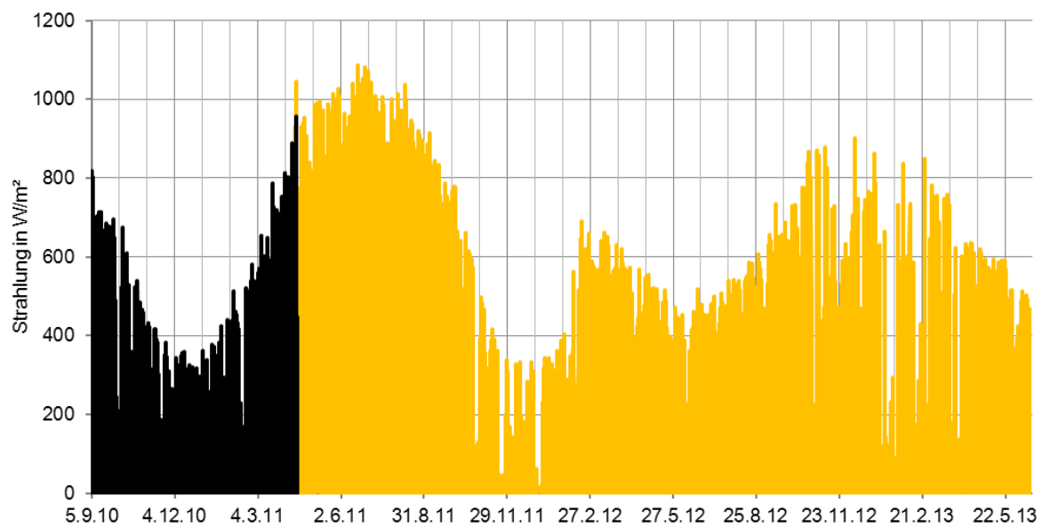
Abb. 46 Jahresgang der Strahlung: Gelb die am Testhaus gemessenen Werte, schwarz die Werte der nahe gelegenen Universitätsmessstation (30-Minuten-Werte); am 8.2.2012 wurde das Sternpyranometer von einer horizontalen in eine vertikale Stellung gebracht
