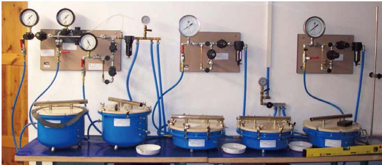
Abb. 35 Druckplattenapparaturen zur Bestimmung der Wasserretention von kapillarporösen Baustoffen
