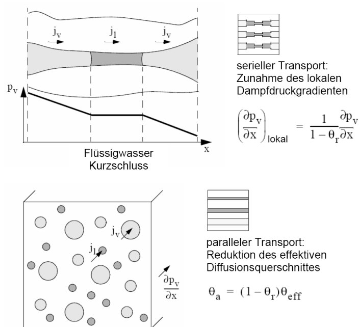
Abb. 40 Mechanismen des Seriell- und Parallelflusses: (oben) Wasserdampfdiffusion mit dem Beitragen der Kondensation, Flüssigwasserfluss und Evaporation an der anderen Seite der lokalen Wasserphase; (unten) Dampfdiffusion mit und ohne Beteiligung der flüssigen Phase jedoch mit Reduktion des effektiven Diffusionsquerschnittes in Form von Kapillarwasser.
