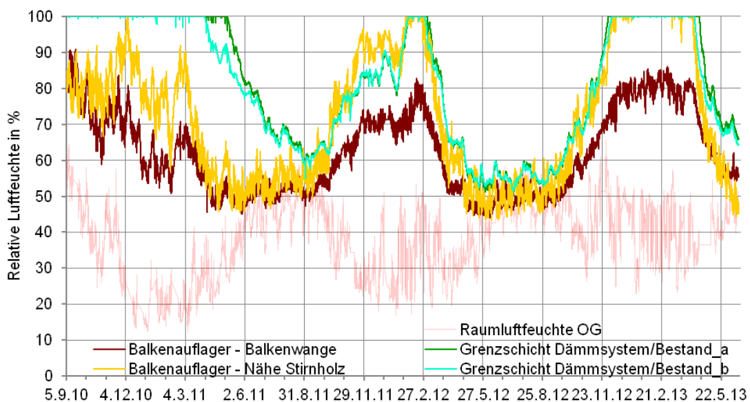
Abb. 77 Stundenwerte der relativen Luftfeuchte an Balken 1: ehemalige Wandoberfläche (grün & hellblau), Balkenwange (braun), neben der Stirnfläche des Balkens (gelb) und Raumlufffeuchte im OG (rot transparent)
