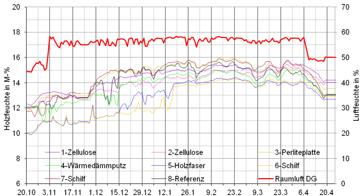
Abb. 94 Holzfeuchte in den Balkenköpfen bzw. an der nassesten Stelle ('HF-St') und Raumlufteuchte im Dachgeschoss vom 20.10. 2012 bis zum 25.4.2013 (Tagesmittelwerte)
