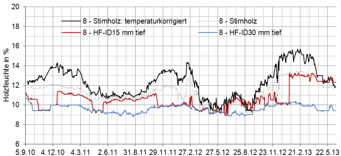
Abb. 70 Gemessene Holzfeuchte an (Referenz-)Balken 8 am Stirnholz und in zwei unterschiedlichen Tiefen (15 und 30 mm) auf der Ebene der Bestands-oberfläche; grau-gestrichelt der nicht-temperaturkorrigierte, tatsächlich gemessene Verlauf der Holzfeuchte am Stirnholz
