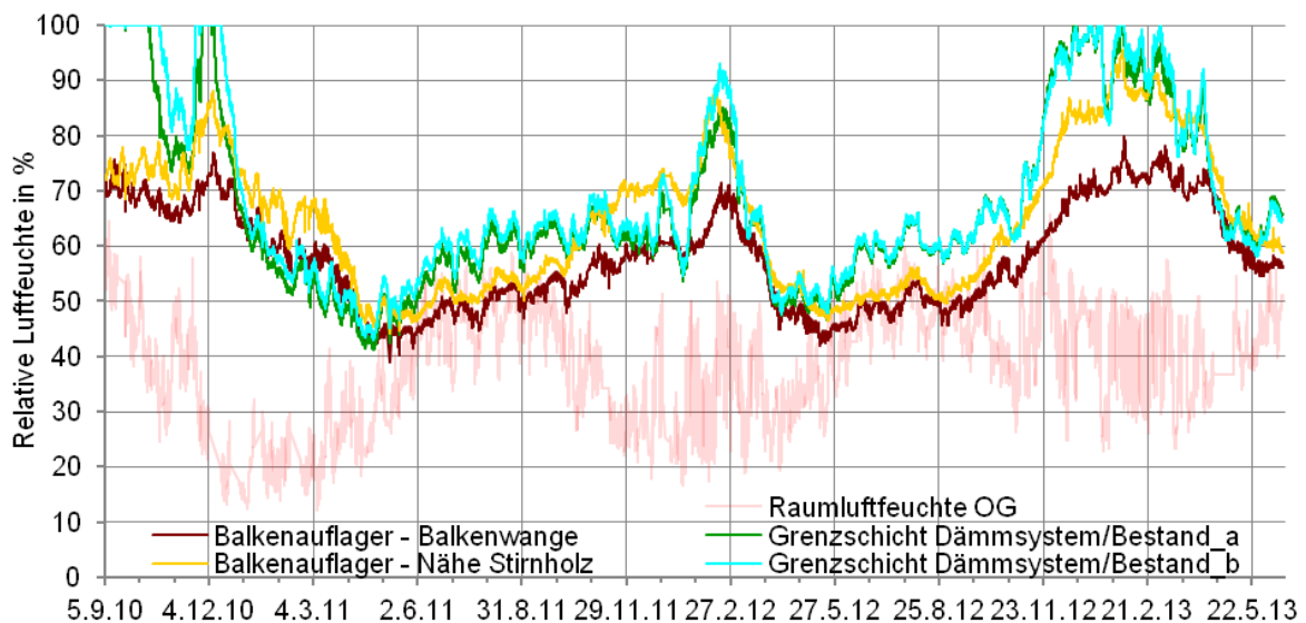
Abb. 85 Stundenwerte der relative Luftfeuchte an Balken 5: ehemalige Wandoberfläche (grün & hellblau), Balkenwange (braun), neben der Stirnfläche des Balkens (gelb) und Raumluftfeuchte im OG (rot transparent)
