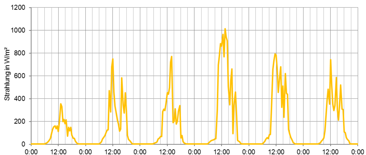
Abb. 47 Verlauf der Globalstrahlung vom 29.7. bis zum 4.8.2011
