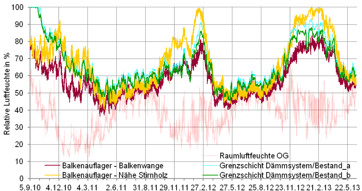
Abb. 81 Stundenwerte der relative Luftfeuchte an Balken 3: ehemalige Wandoberfläche (grün & hellblau), Balkenwange (braun), neben der Stirnfläche des Balkens (gelb) und Raumluftfeuchte im OG (rot transparent)
