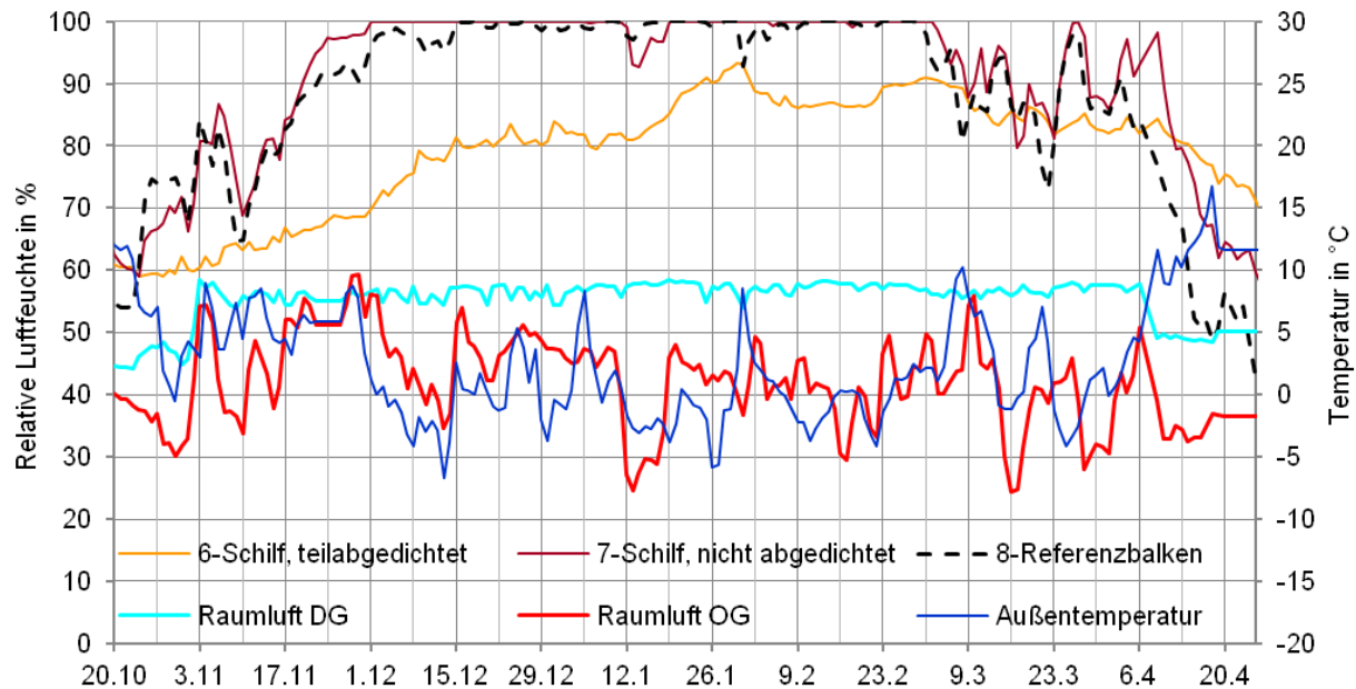
Abb. 92 Tageswerte der Luftfeuchte in Stirnholznähe (BA-St) 6 bis 8 und im Dach-(hellblau) - und Obergeschoss sowie Tageswerte der Außentemperatur (blau) vom 20.10. 2012 bis zum 25.4.2013
