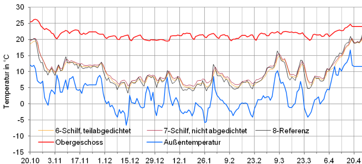
Abb. 95 Temperatur am Ende der Balkenauftragertaschen 6 bis 8 sowie Temperatur im Obergeschoss und Außenbereich vom 20.10. 2012 bis zum 25.4.2013 (Tagesmittelwerte)
